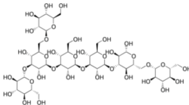
\beta -glucan
